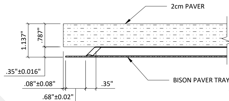
D1 BISON PAVER TRAY/2cm PAVER WIND SYSTEM EDGE DETAIL SCALE: 6" = 1'-0"
