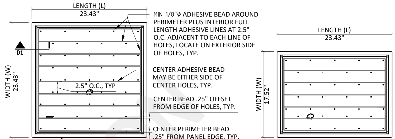
T1 BISON 24 x 24 PAVER TRAY - TOP VIEW SCALE: 1" = 1'-0"
